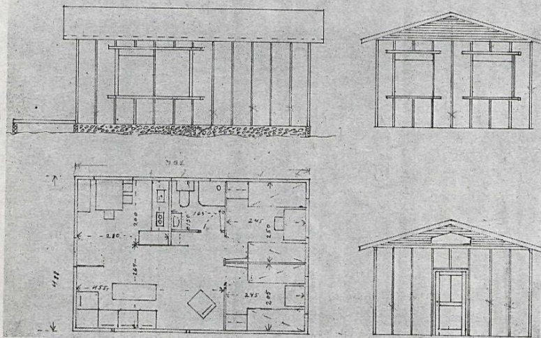
Þessir uppdrættir sýna hús í líkingu við það, sem talað er um í greininni. Í þessu húsi, sem er 35 fermetrar, eru tvö svefnherbergi, bað, eldhús og stofa.
