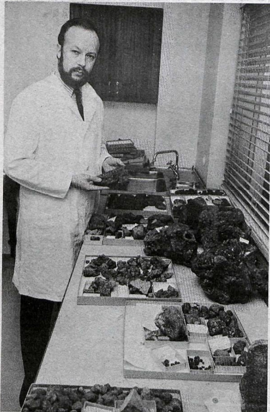
Sveinn Jakobsson handleikur blágrýtissýni, sem tekin voru neðansjárvar úr Kolbeinseyjarhryggnum í haust.
