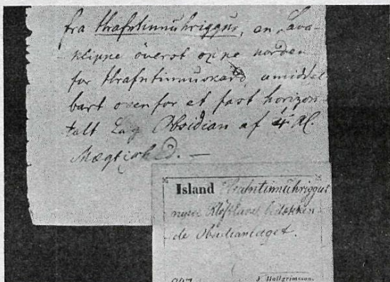
Merking á einu sýnishornanna í jarðfræðisafninu í Kaupmannahöfn, skráð með hendi Jónasar Hallgrímssonar. Tímamyndir Róbert.
