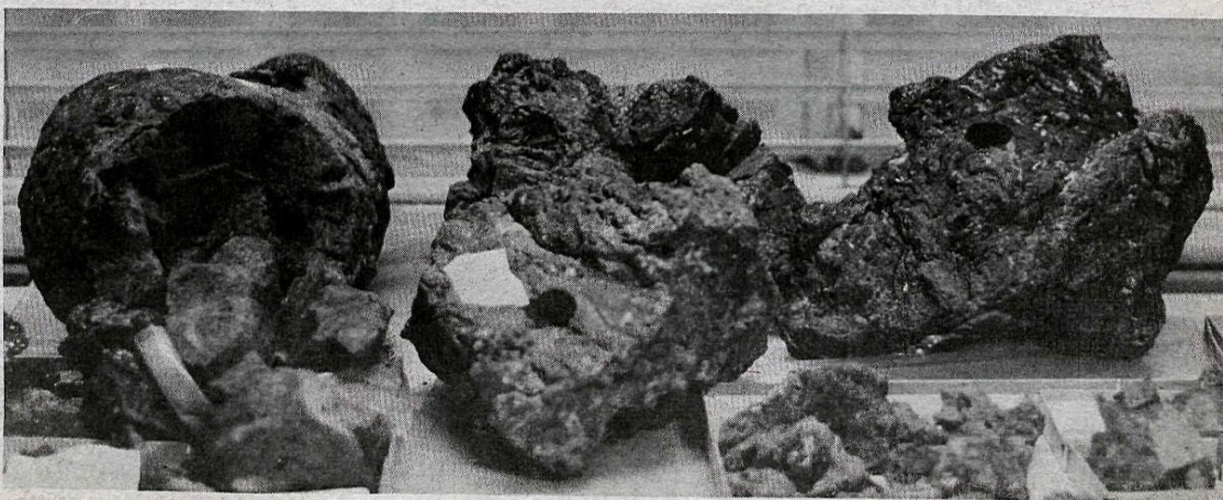
Botnsýni úr neðansjárvarhryggnum norðan Kolbeinseyjar, sem vísindamenn á rannsóknaskipinu „Lynch” tóku.
