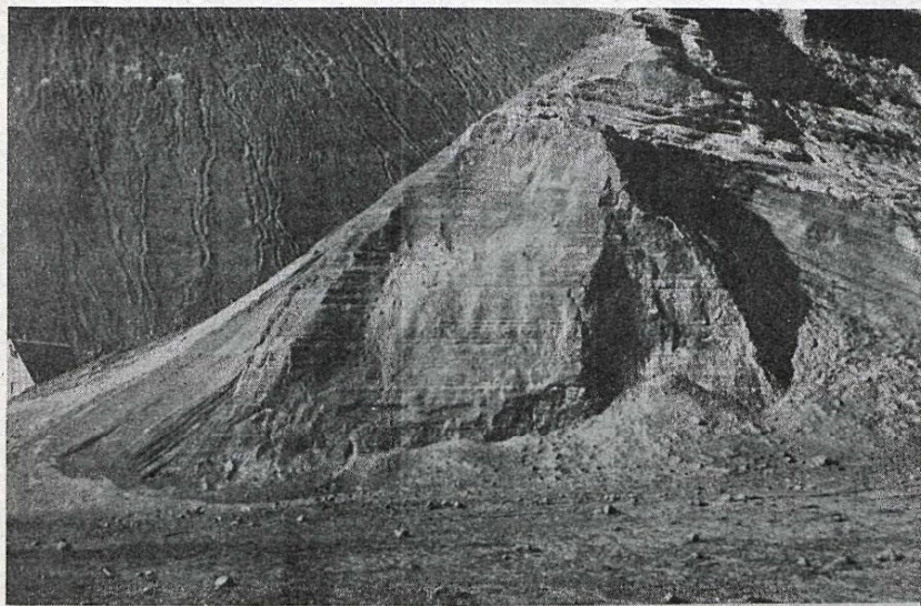
Landslag á norðurstönd Surtseyjar.
