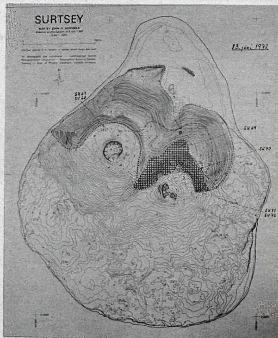
Rúðstríkaði hlutinn á þessu korti sýnir móbergssvæðið í Surtsey.
