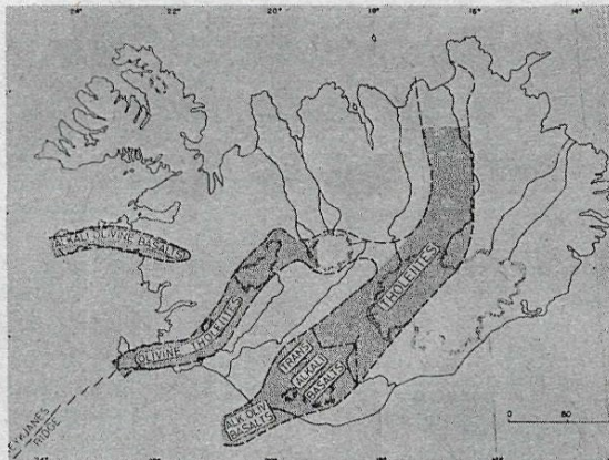
Þetta kort sýnir dreifingu hinna ýmsu gerða blágrýtishrauna á gosbeltum landsins.
